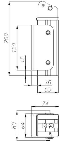
Mocowanie do podłoża naturalnego
